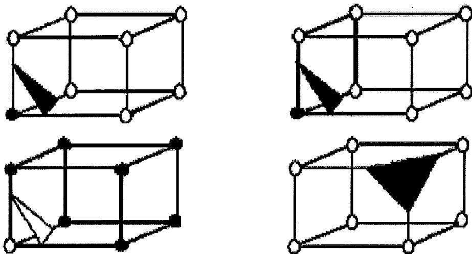
Figura 4.4: Simetrias: complementar inversa(à esquerda); rotacional (à direita).
