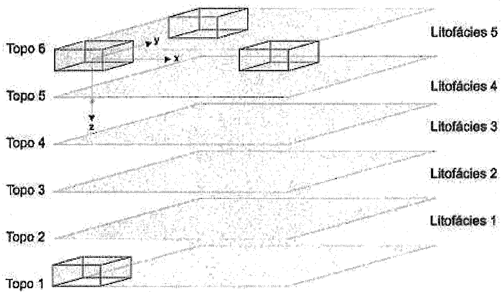
Figura 5.2: Geração de voxels do volume litofaciológico.
