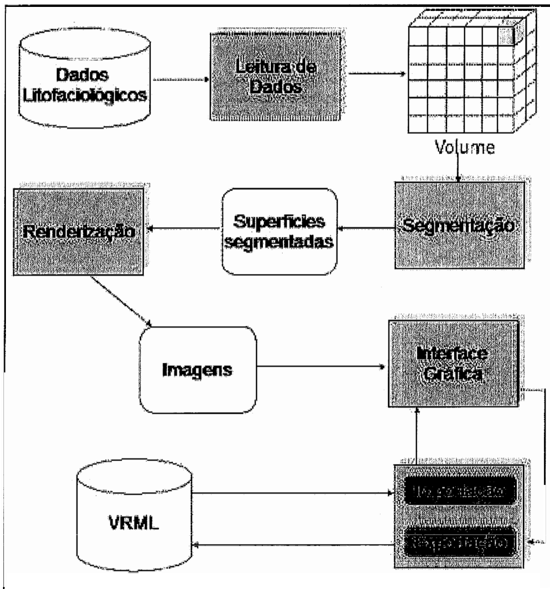
Figura 4.1: Arquitetura do Sistema.
