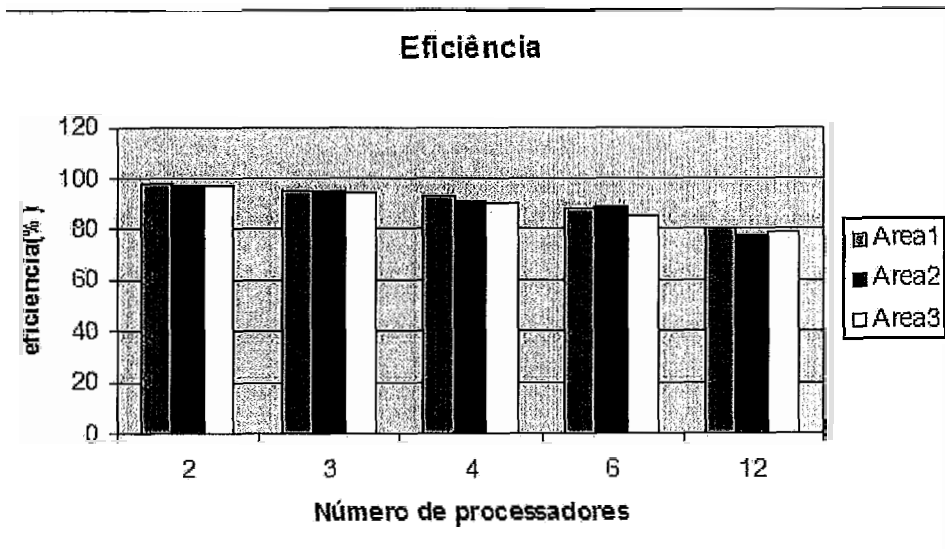
Figura 5.7: Eficiências obtidas para as áreas 1,2 e 3.
