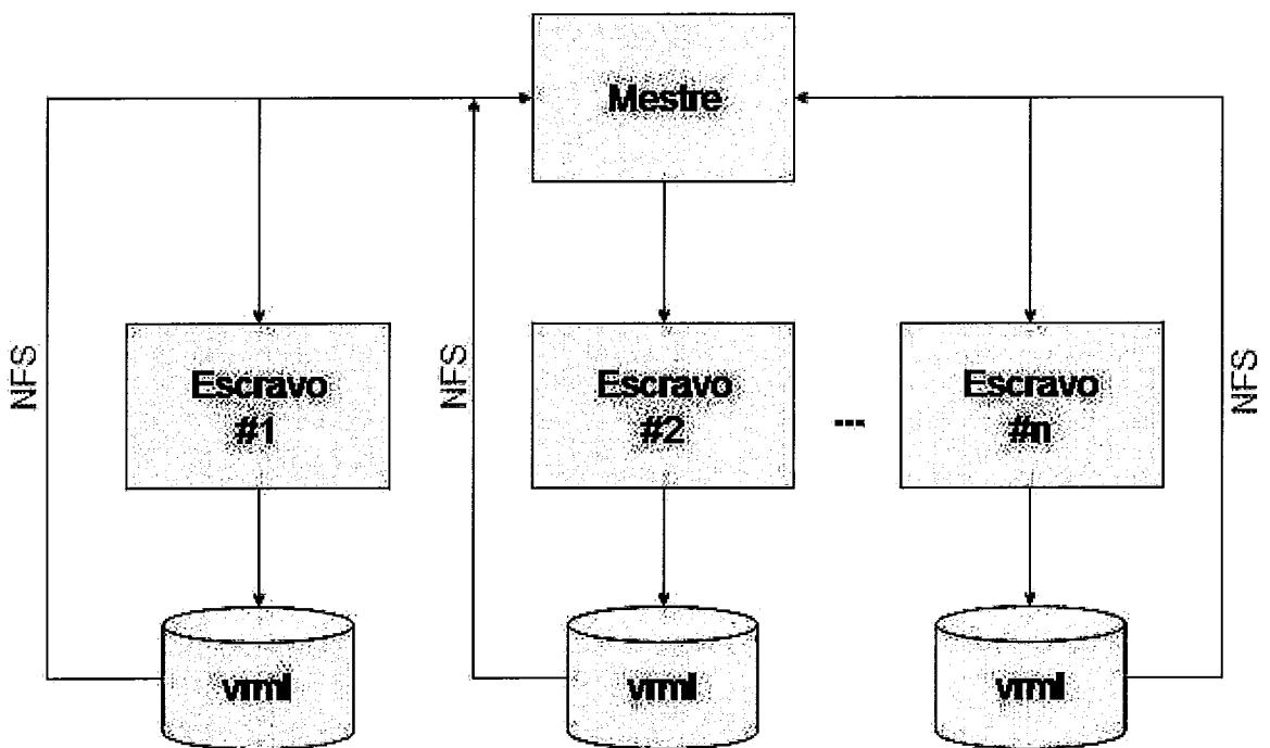
Figura 4.9: Arquitetura do Sistema Paralelo.
