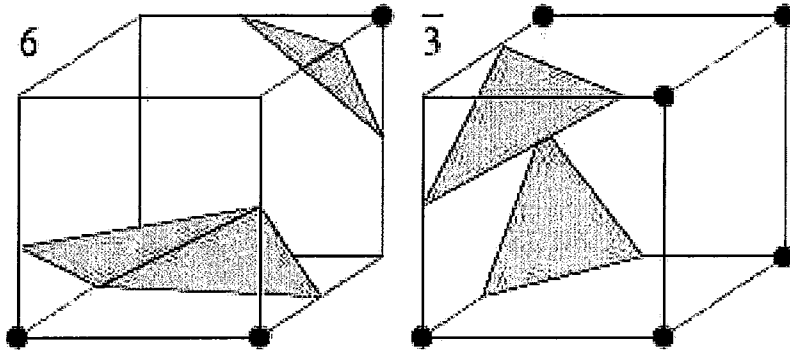
Figura 4.6: Buraco na face compartilhada entre dois voxels.
