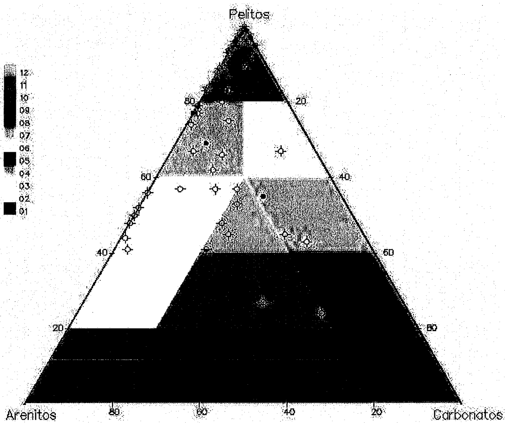
Figura 2.4: Esquema arenitos-pelitos-carbonatos [9].
